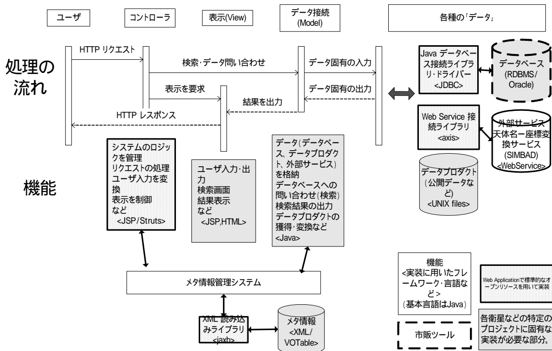
図 1 開発中のデータ検索・転送システムのソフトウェア構成
