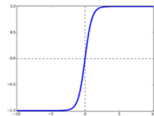
tanh
