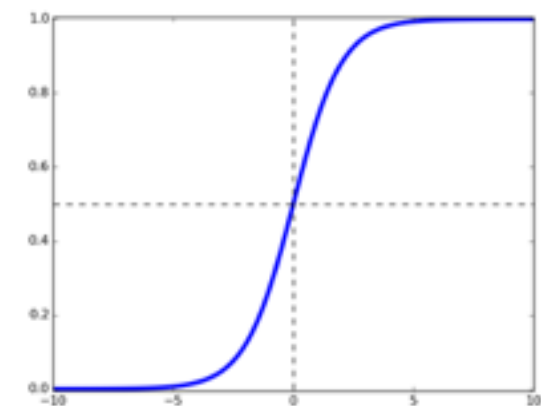
sigmoid
